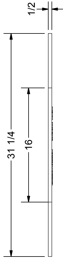
SECTION A-A
