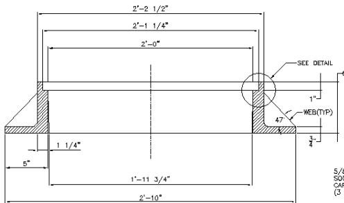
MANHOLE RING - SECTION
